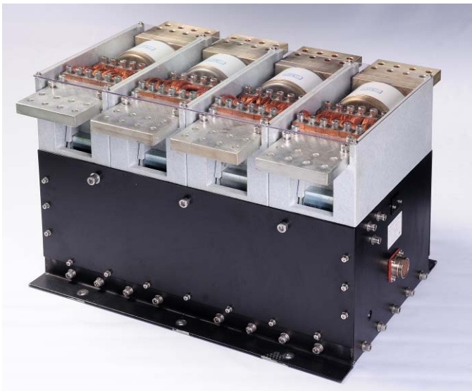
CKJ11-3000 型交流真空接触器
